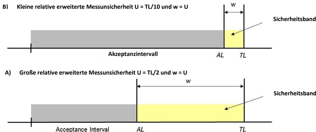
Abbildung 6: Akzeptanzintervall für einen Fall, in dem die erweiterte Messunsicherheit bei gleicher Toleranzgrenze TL im Vergleich zur Toleranz klein ist A) und groß ist B). Ein großes Sicherheitsband verengt die Verteilungsfunktion der akzeptierten Gegenstände.
