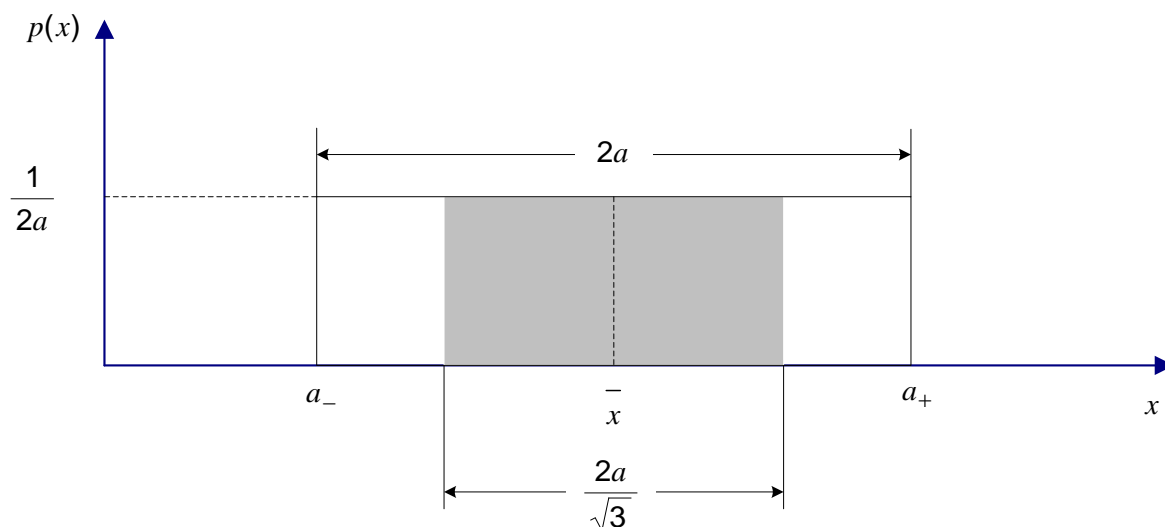
Bild 2 - Rechteckförmige symmetrische Wahrscheinlichkeitsverteilung p(x) der Schätzung x einer Eingangsgröße X
