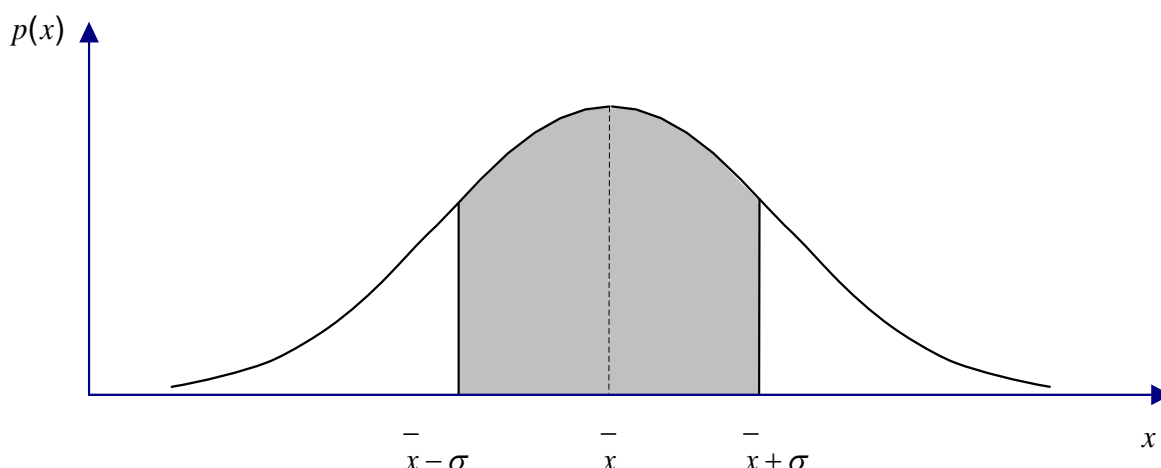
Bild 1 - Normal Wahrscheinlichkeitsverteilung p(x) einer stetigen Zufallsvariablen x
